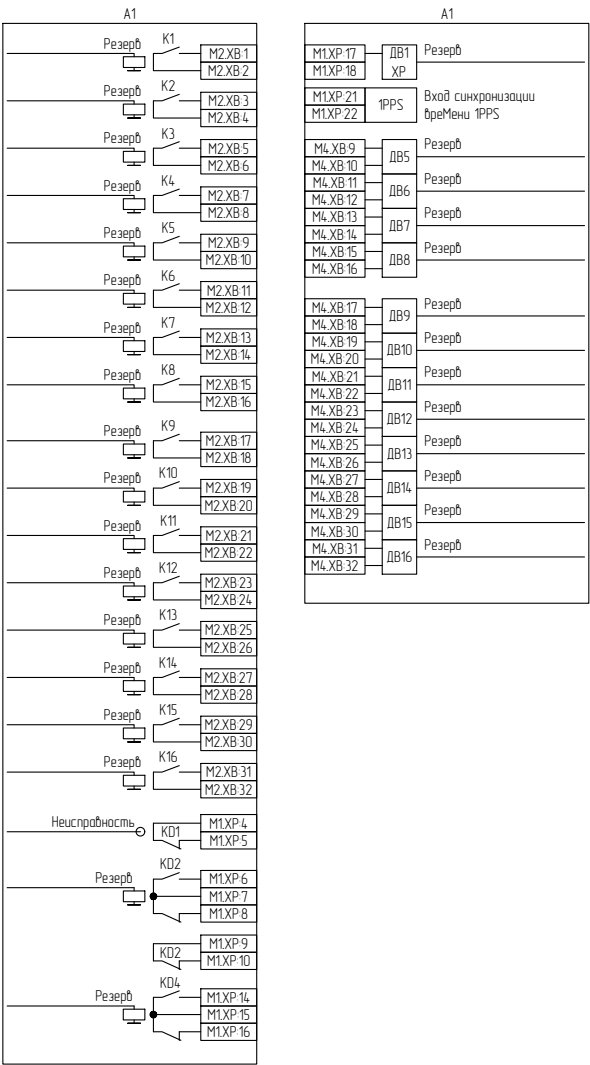
Рисунок Г.3 – Схема электрическая принципиальная (часть 3)
